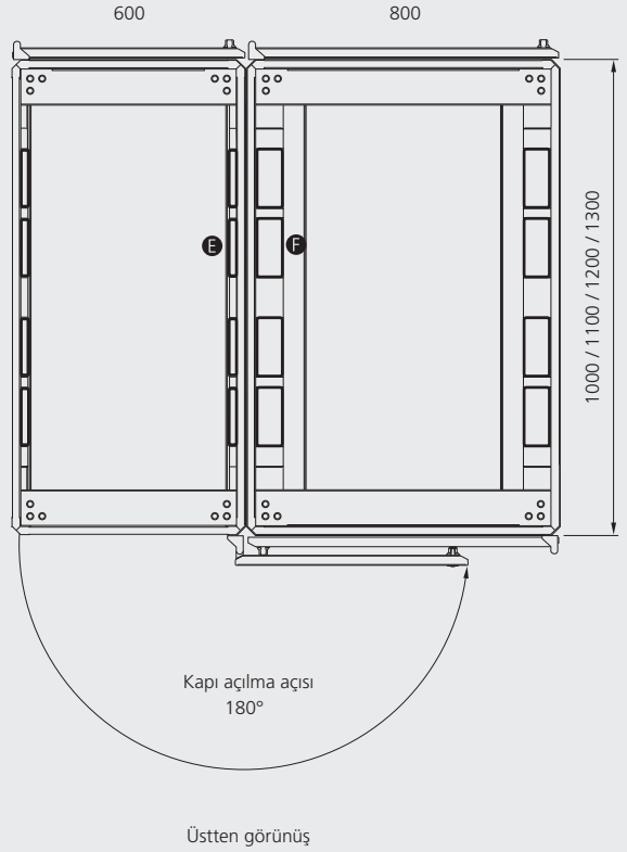
Kabinet Geniřlięi
