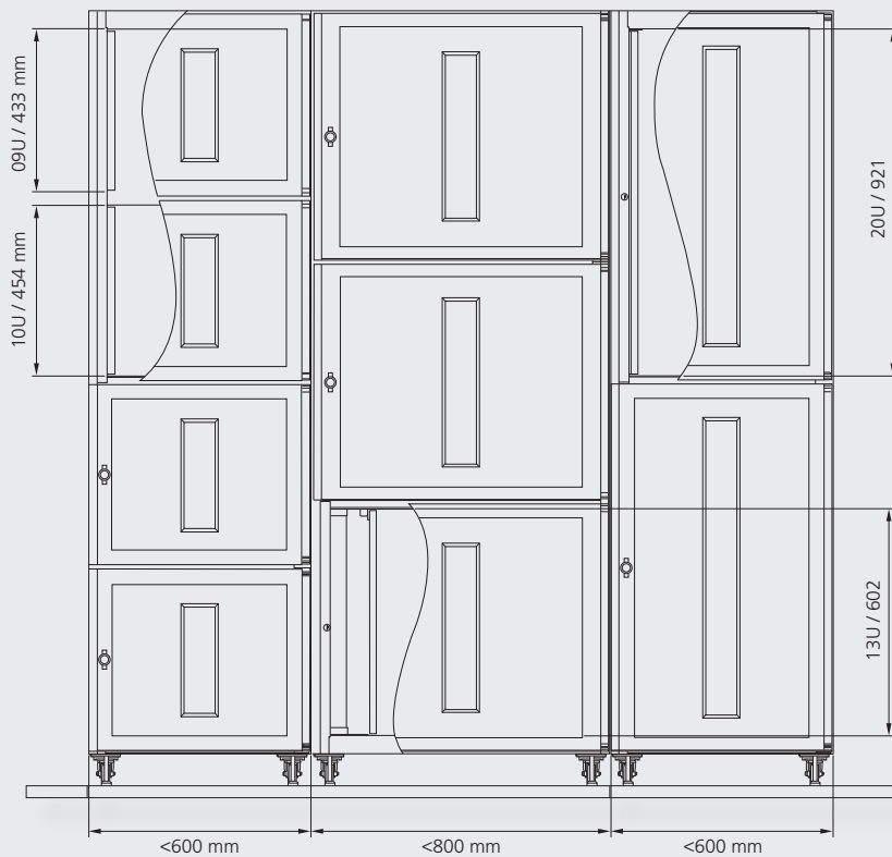
Kabinet Yüksekliği 42U
