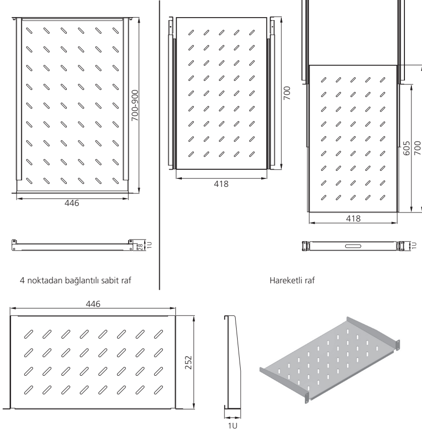
Tek taraftan bağlantılı sabit raf
