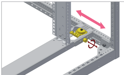
Sonsuz vidalı tip - sürekli, adımsız ayarlanabilir
