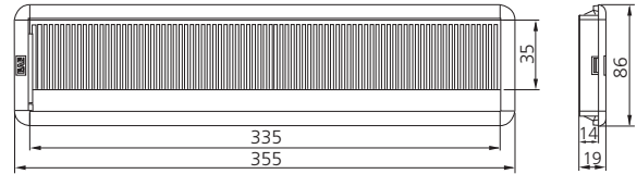
KP CO 01 B Fırçalı Kablo Giriş Modülü
