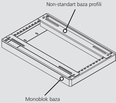
Monoblok baza
