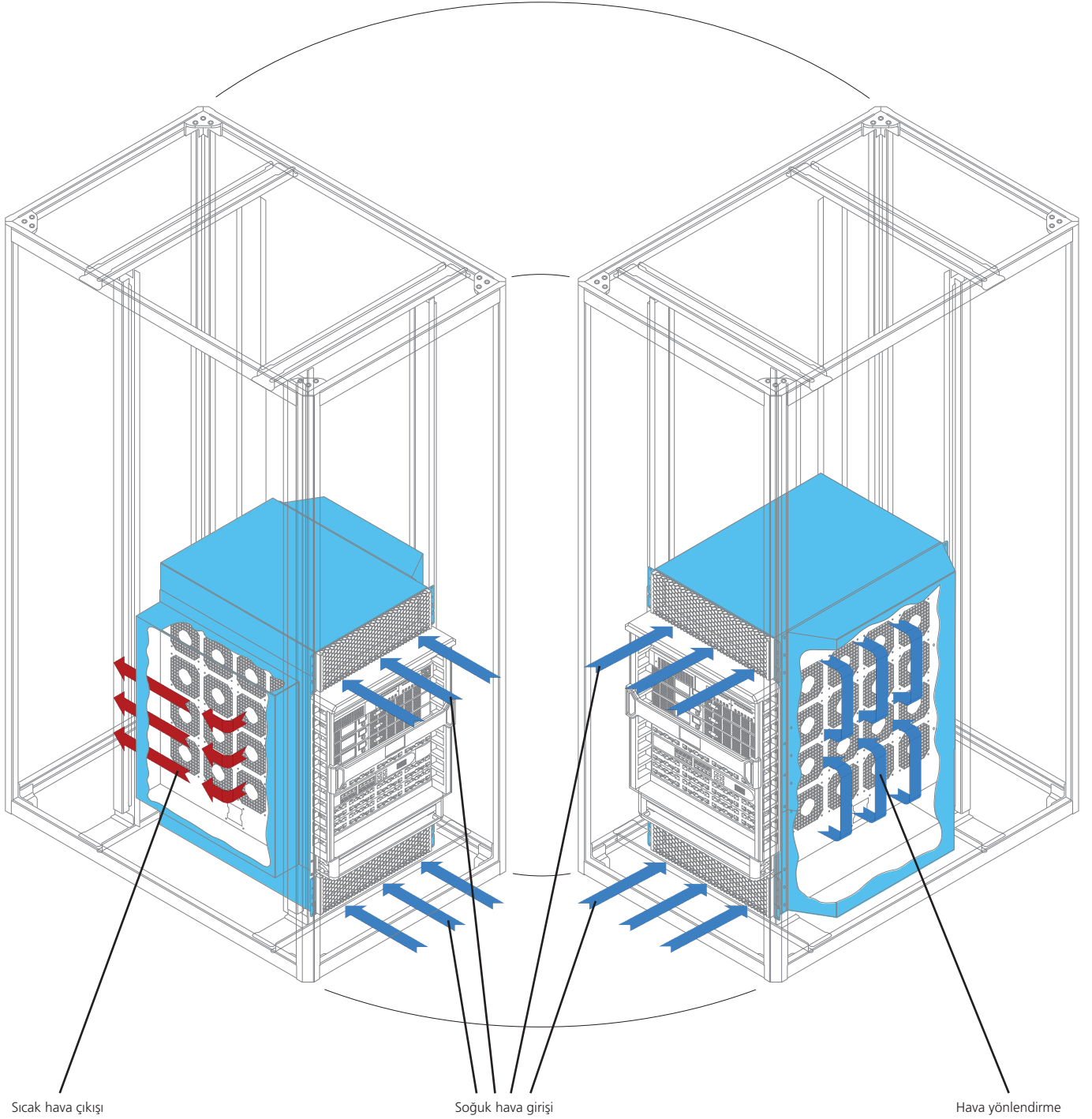
Örnek 14U Cisco Nexus 7009 Switch uygulaması
