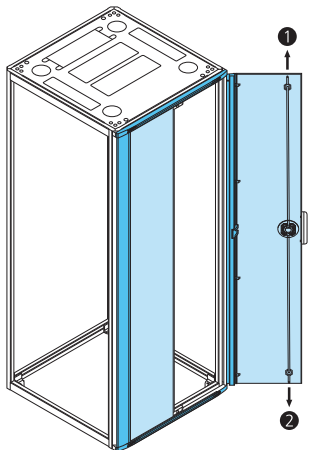
2 noktadan kilitleme
