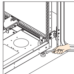
Dışarıdan ayar
