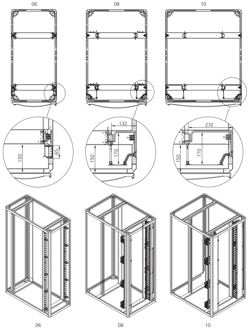
Dikey Kablo Düzenleyici
