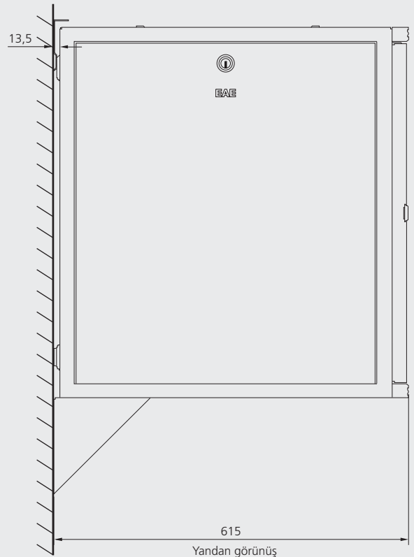
Yandan görünüş
