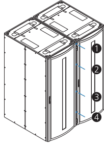
Kabinet Birleştirme Kiti / Ön - Arka
