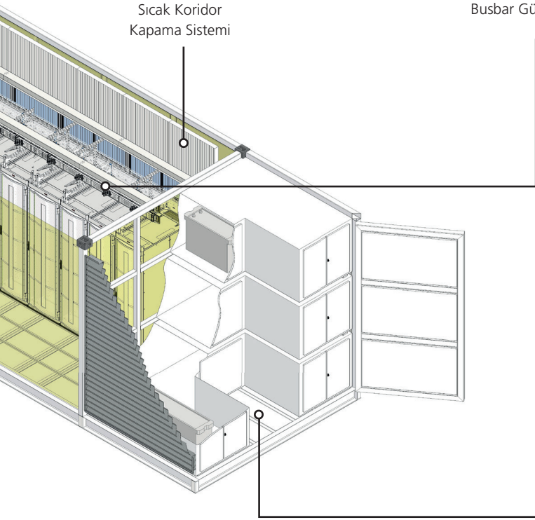
Soğutma Sistemi Teknik Odası
