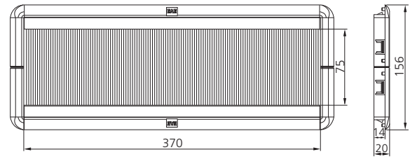
KP CO 02 B Fırçalı Kablo Giriş Modülü
