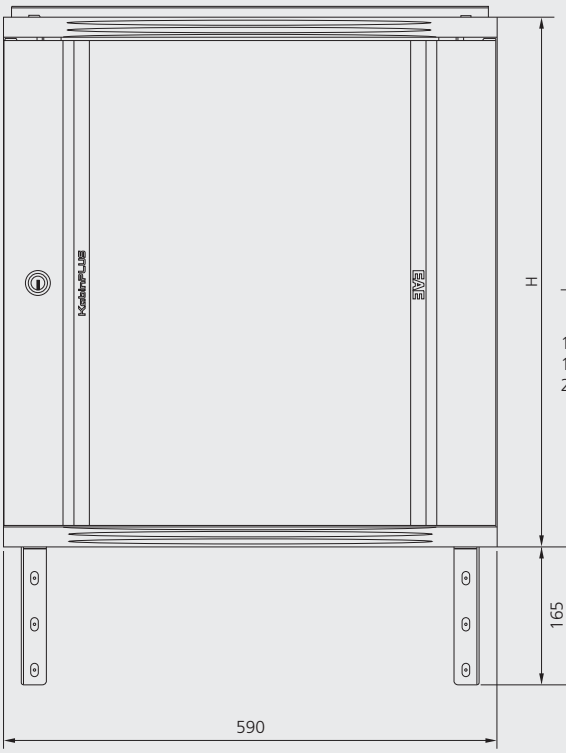
Önden görünüş
