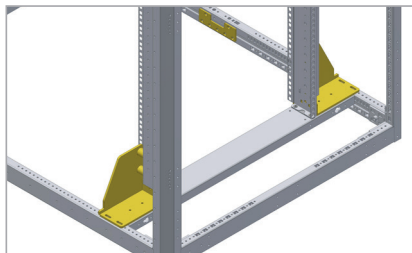
Sismik taşıyıcı alternatifi (sayfa 98'e bakınız)
