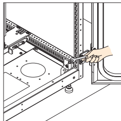
İçeriden ayar
