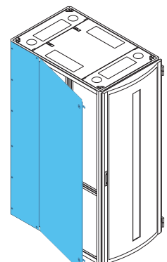
Koridor başı yan kapak
