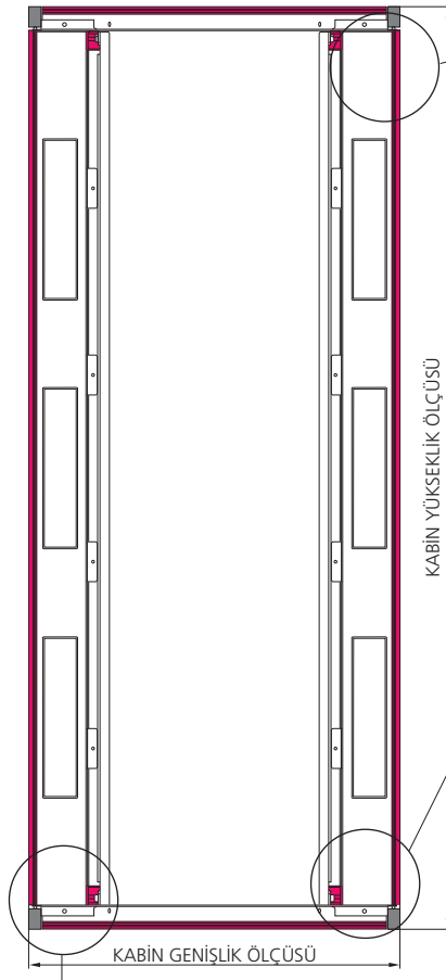
Dikey Hava Kapama Grubu
