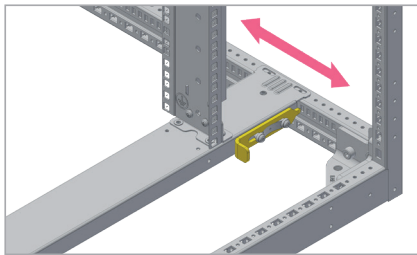
Sürgülü tip - 10 mm adımlarla ayarlanabilir
