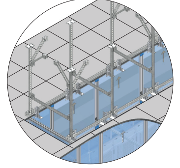
Sismik Askı Tasarımı
