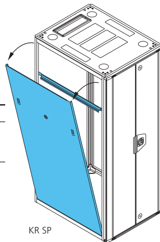
Çıkarılabilir Yan Kapak
