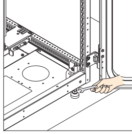
Dışarıdan ayar
